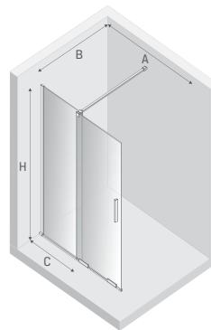
Možnosť 1 Kolmá vzpera Možnosť 1 Kolmá vzpěra Opțiunea 1 Suport perpendicular Opció 1 - Merőleges támaszték
